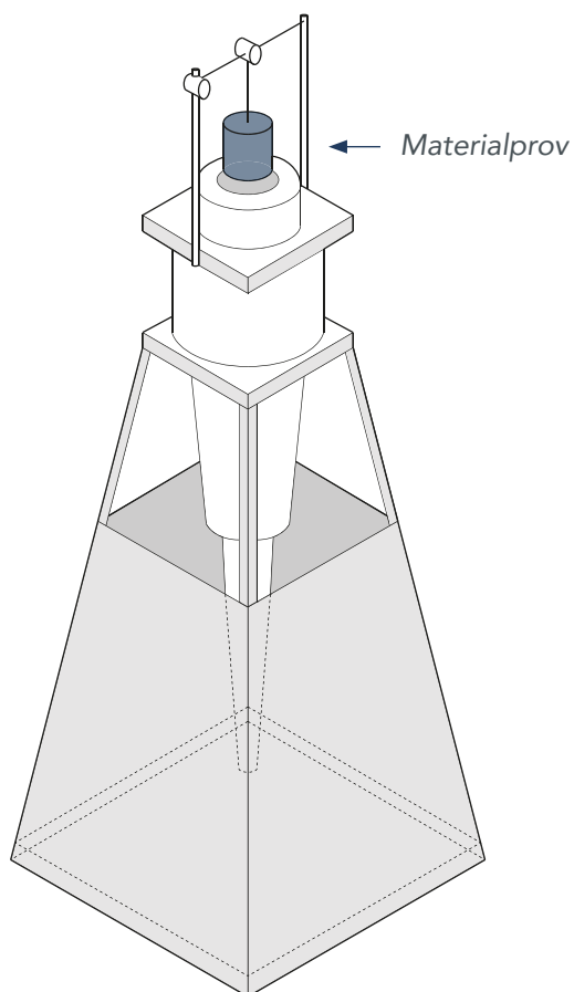
Icke-brännbarhetstest
