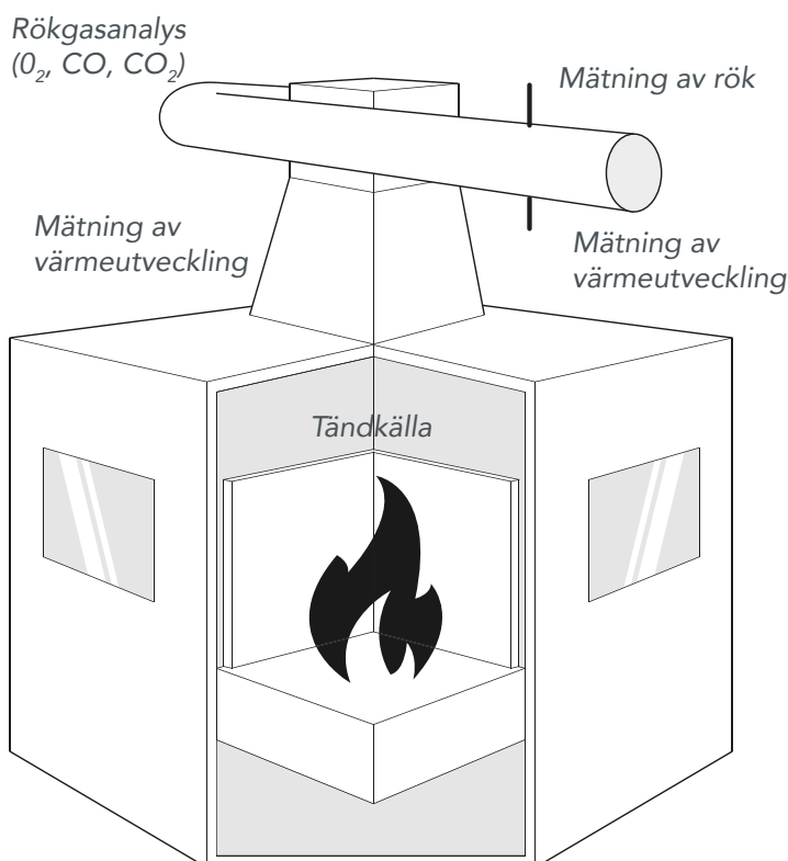
SBI test
