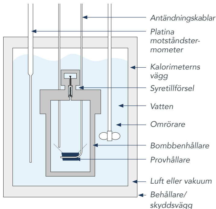
Kalorimeter för syrgasbomb
