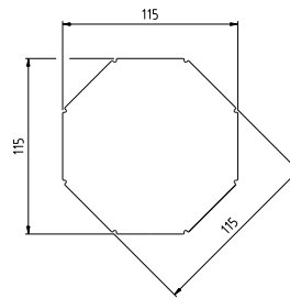
DETALJ: STOLPE
