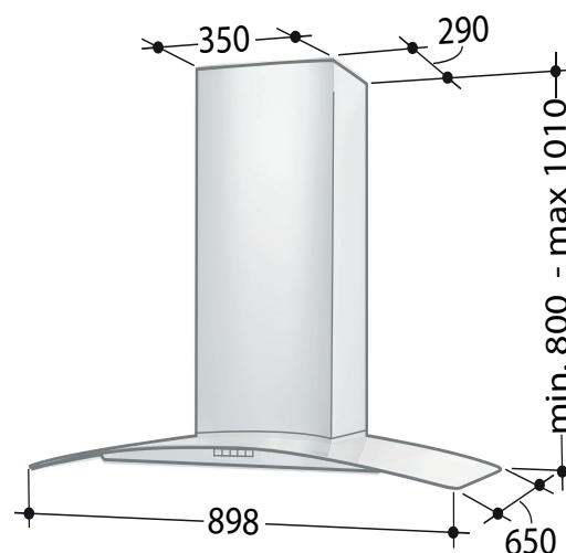
Måttskiss - 774 frihängd
