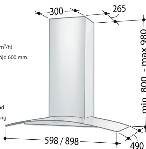
Måttskiss - 764 väggmonterad
