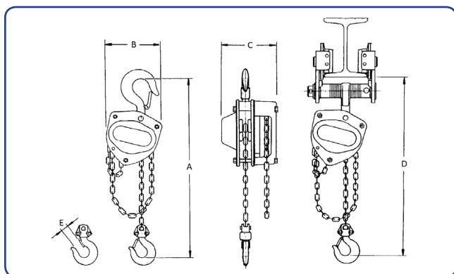
Måttskiss KITO Mighty CB
