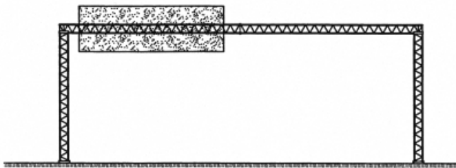
2-bent portal
