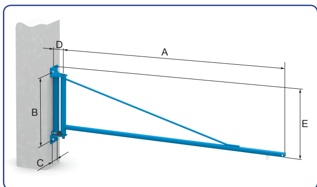
Måttskiss FREJ Väggsvingkran
