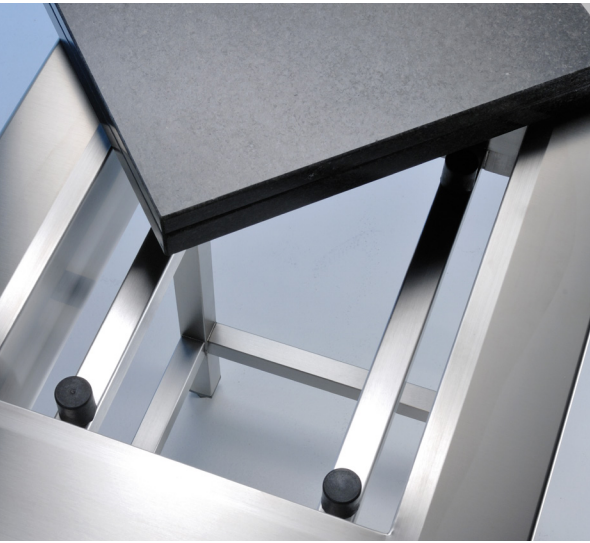
Wiegetisch inkl. Anti-Vibrations-Blöcke Weighing table incl. anti-vibration bearings
