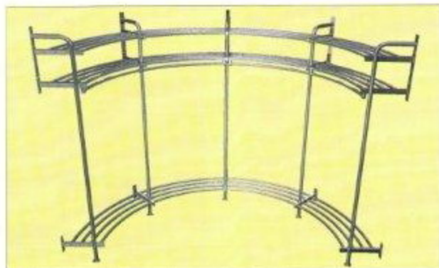
Fig 13. Klädställ nr 212 BVK med fast skohylla och rullbockade hyllor
