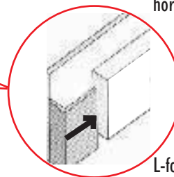
Invändig hörnprofil
